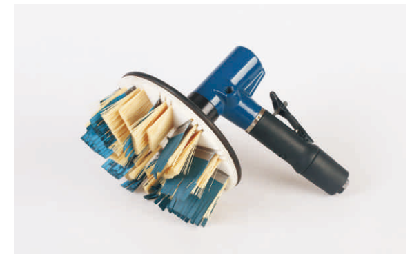
异形盘式打磨机 / Portable profile disk sander
